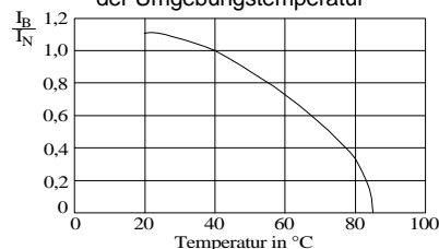
Zulässiger Betriebsstrom in Abhängigkeit der Umgebungstemperatur
